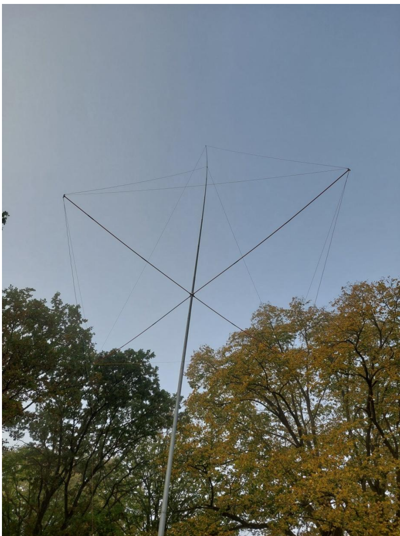
Antena rombowa SQ1GU
