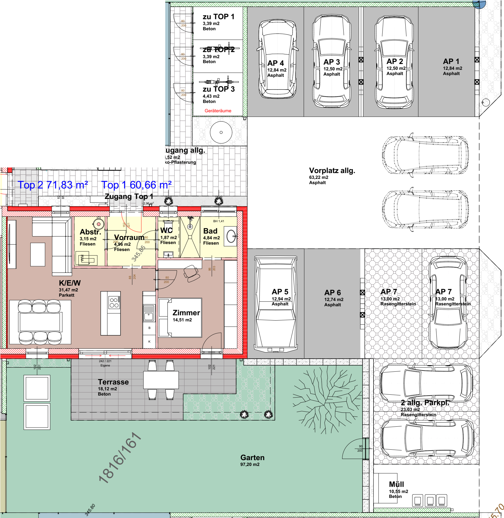
Erdgeschoss
