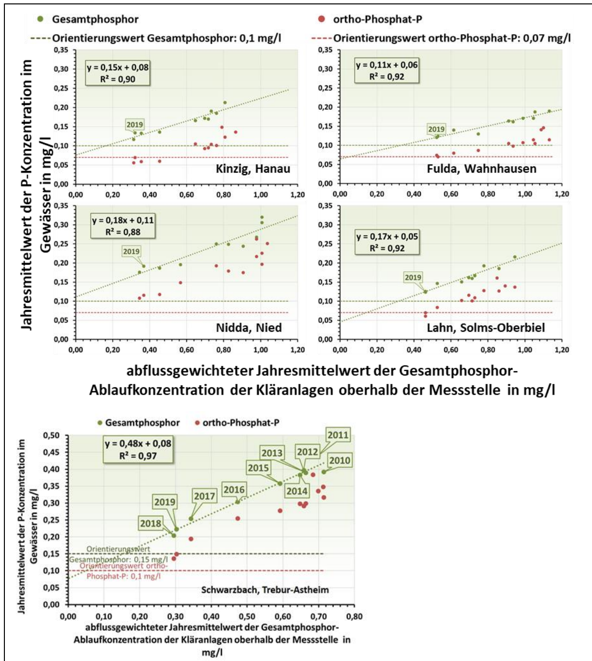
Abbildung 18: Abhängigkeiten zwischen Gewässerkonzentrationen und Ablaufkonzentrationen der entsprechenden Kläranlagen an hessischen Flüssen (Quelle: HESSISCHES LANDESAMT FÜR NATURSCHUTZ, UMWELT UND GEOLOGIE)
