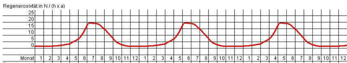
Abbildung 27: Beispielhafte Jahresverteilung der Regenerosität, aus „Bodenerosion durch Wasser“, Landwirtschaftskammer NRW, 2007
