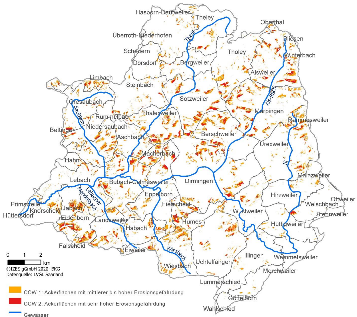
Abbildung 12 CCW 2018 Erosionsklassen im Einzugsgebiet von Theel und Ill (IZES, 2020)
