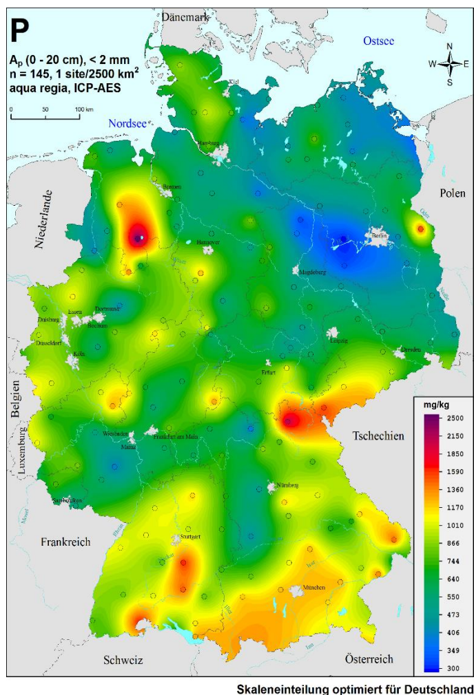
Abbildung 9: Phosphor in deutschen Ackerböden; Daten aus GEMAS-Projekt, Geologisches Jahrbuch B 102 von 2014, Dr. Birke, Bundesanstalt für Geowissenschaften und Rohstoffe
