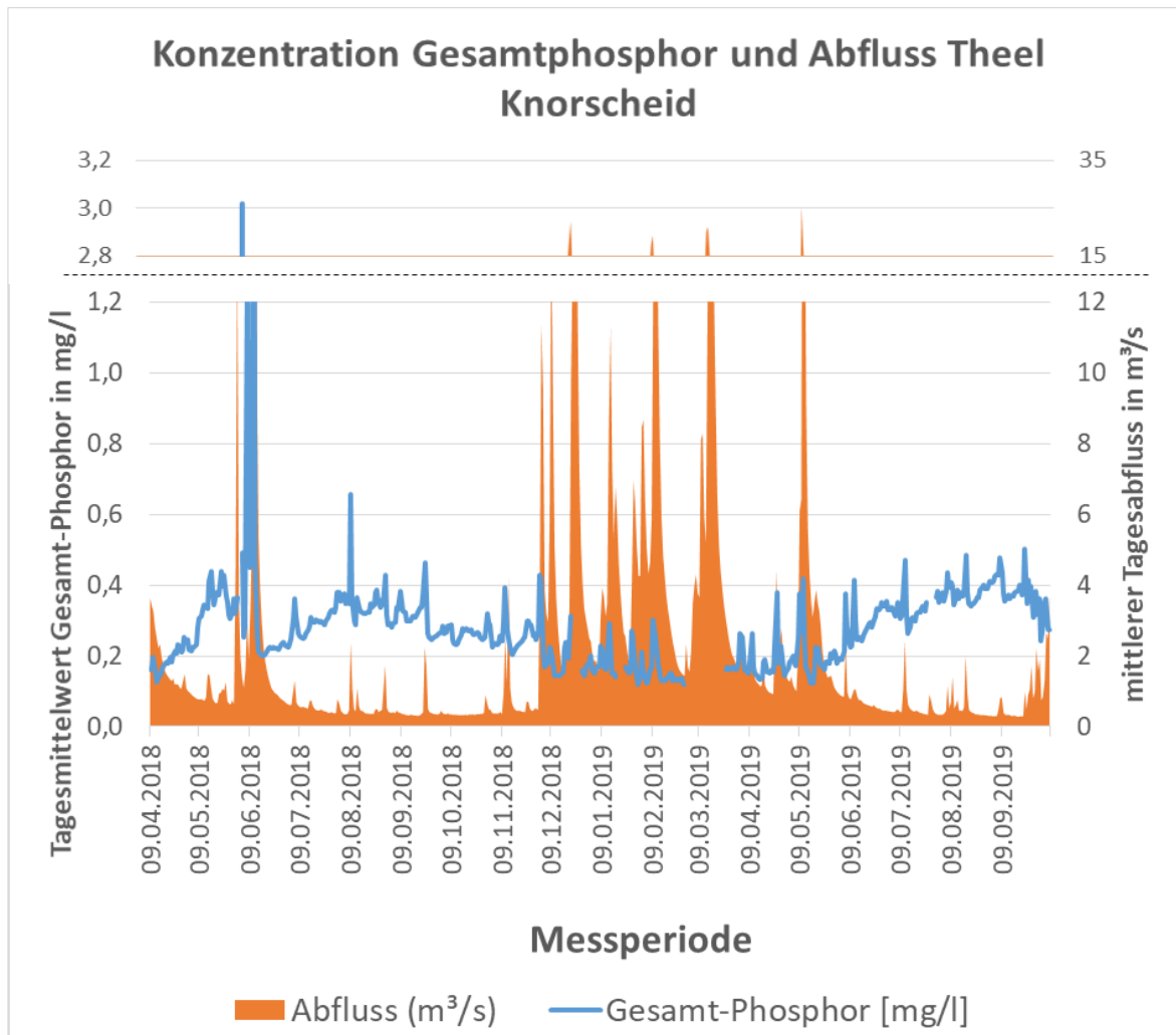
Abbildung 22: Konzentration von Gesamtphosphor als Tagesmittelwerte aus den online-Messungen der UdS an der Theel im Vergleich zum Abfluss der Theel
