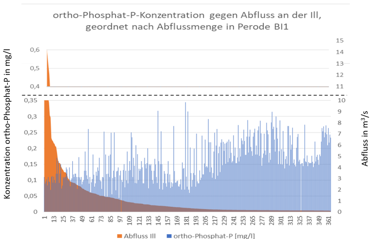
Abbildung 23: ortho-Phosphat-P-Konzentrationen im Vergleich zum Abfluss an der III (BI1), Daten geordnet nach Höhe des Abflusses, Abfluss bei 10 m³/s gekappt
