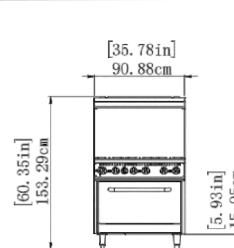
PFFSO-36-J
