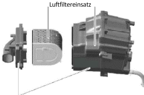
Luftfiltergehäuse
