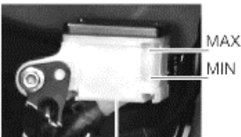
Sichtfenster für die hintere Bremsflüssigkeit
