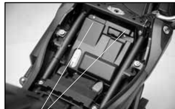
Schrauben zur Öffnung des Sitzes
