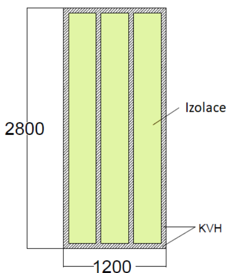
Příčný řez
