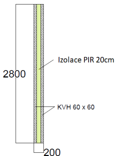
Podélný řez
