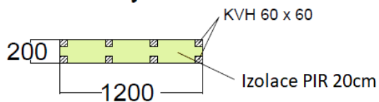
Příčný řez
