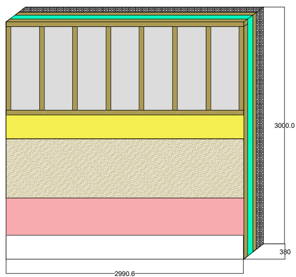
Přední pohled
